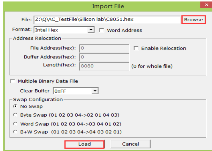
图 5 烧录档案选择界面
