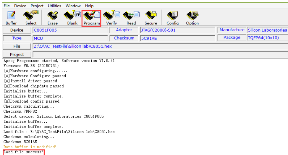
图 6 烧录档案加载成功后显示的界面
